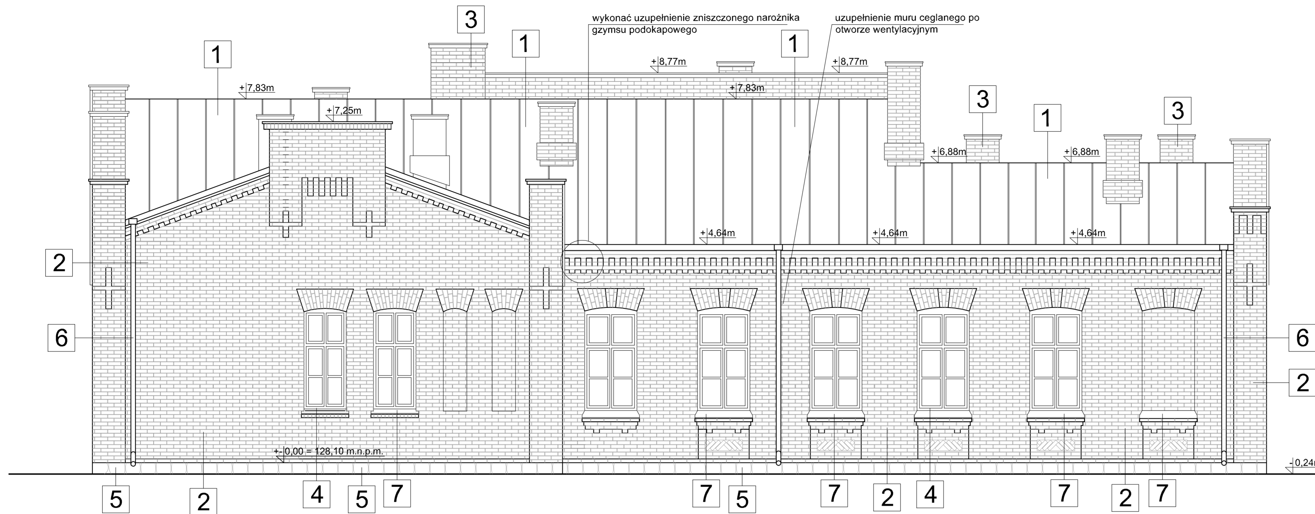
ELEWACJA POŁUDNIOWO-ZACHODNIA, SKALA 1:50 / DZIEŚIĘCIOOSIOWA, NIESYMETRYCZNA, ROZCZŁONKOWANA /
