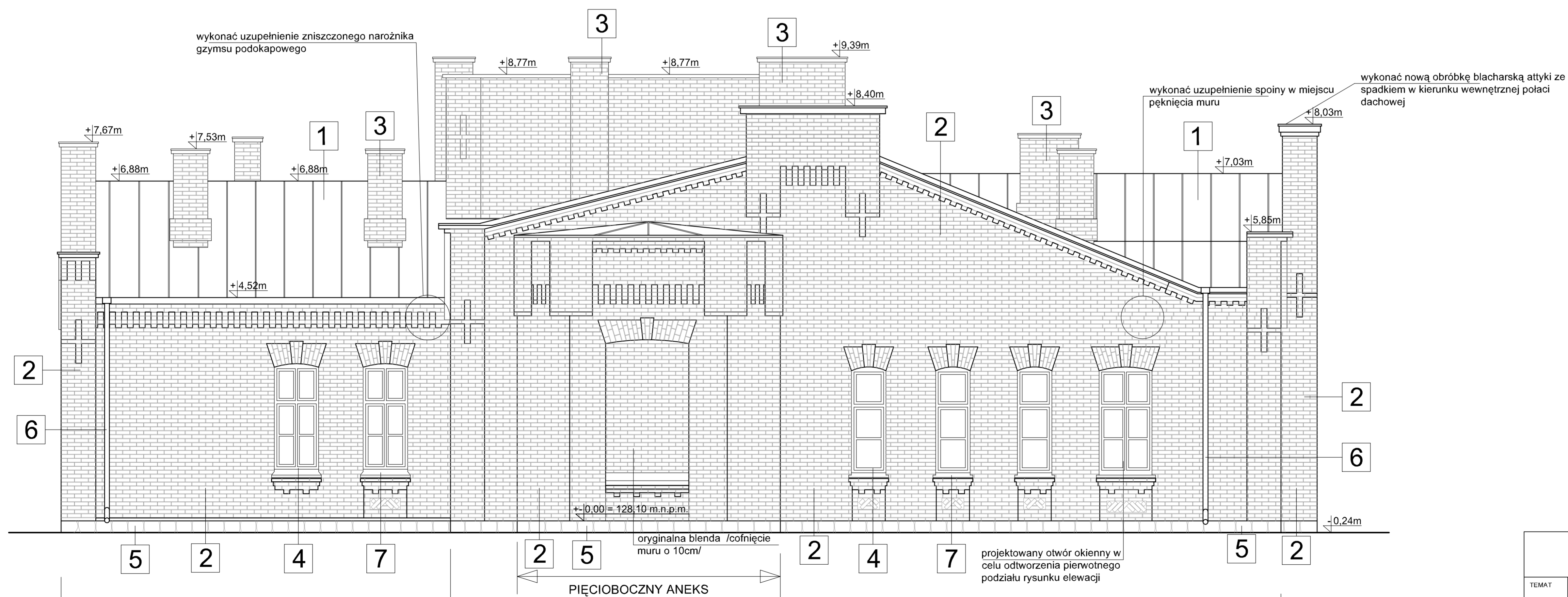
ELEWACJA PÓŁNOCNO-WSCHODNIA, SKALA 1:50
